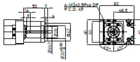
Motor Adaptor Flange F1
